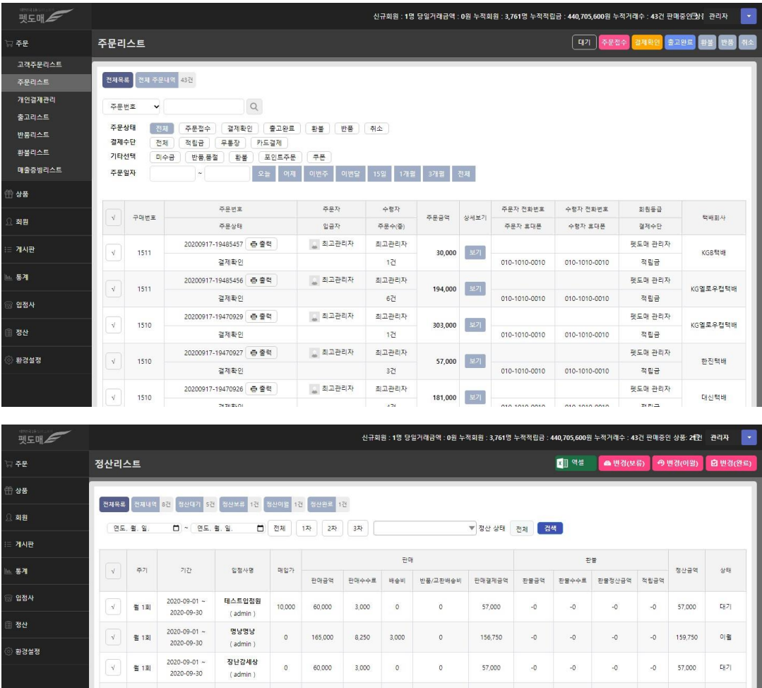
고객 주문 리스트 각 입점사별 주문번호 개별생성 주문서 출력 기능
